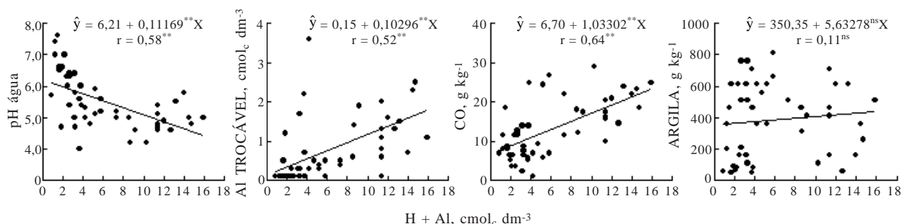
Figura 2. Correlação linear simples entre pH em água, Al trocável ( \text{Al}^{3+} ), carbono orgânico (CO) e teor de argila e a acidez potencial (H + Al). (** significativo a 1% pelo teste de t).
