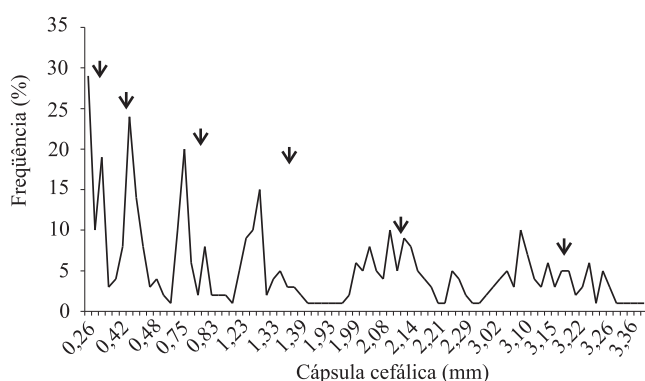
Figura 1. Frequência das medições das cápsulas cefálicas de Agrotis ipsilon durante o desenvolvimento larval em dieta artificial. Temperatura: 26 \pm 1^\circ\text{C} ; umidade relativa do ar: 70 \pm 10\% ; fotófase: 14 horas. As setas indicam os ínstaes.
