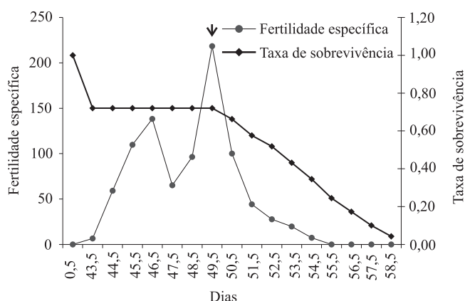
Figura 2. Relação entre fertilidade específica ( m_x ) e taxa de sobrevivência ( l_x ) de Agrotis ipsilon criada em dieta artificial. A seta indica a taxa máxima de aumento. Temperatura: 26 \pm 1^\circ\text{C} ; umidade relativa do ar: 70 \pm 10\% ; fotófase: 14 horas.
