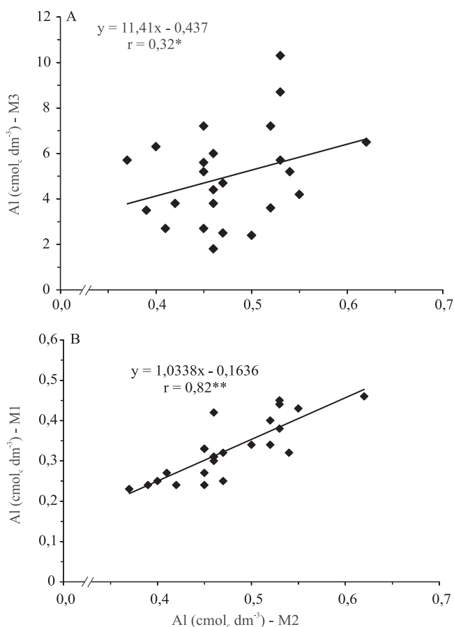
Figura 2. Correlação linear simples (r): A, entre os teores de Al extraídos com KCl e quantificados por espectrofotômetro de absorção atômica com forno de grafite (GF-AAE) (M2), e os extraídos com KCl e quantificados por titulação com NaOH (M3); e B, entre os teores de Al extraídos por KCl e quantificados por GF-AAE (M2), e os extraídos por \text{Ca}(\text{OAc}_2) e quantificados por GF-AAE (M1). ** e * Significativo pelo teste t, a 1 e 5% de probabilidade, respectivamente.
