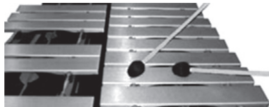
Ex.18: Ataque sobre a região do nó com a baqueta apoiada no centro da lâmina.
