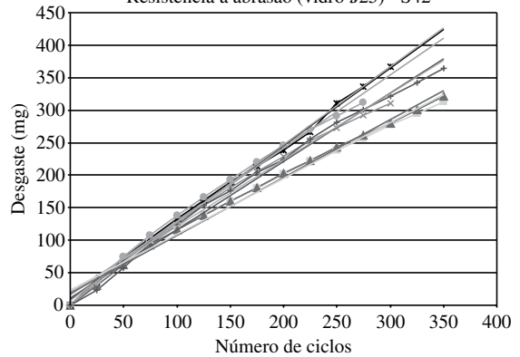
Resistência à abrasão (vidro #25) - S42
