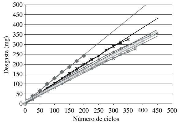
Resistência à abrasão (vidro #00) - S42
