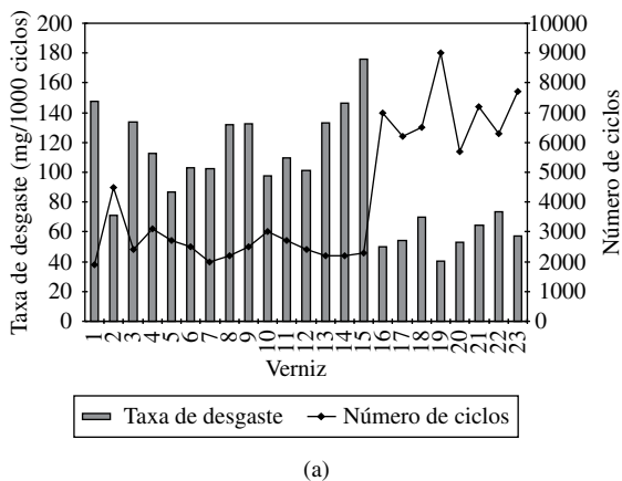
Figura 4. Gráficos de verniz x taxa de desgaste x número de ciclos para os ensaios com a) CS-17; e b) S-42.
