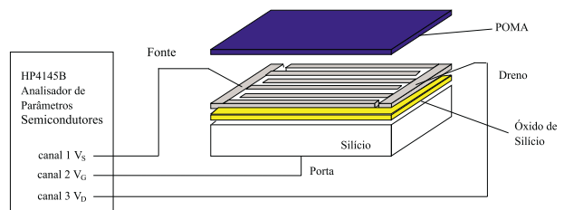
Figura 2 - Esquema da montagem do transistor.
