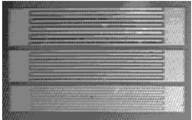
Figura 3 - Foto do transistor a base de POMA
