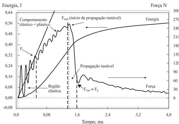
Figura 4. Diagrama esquemático típico de energia de impacto E(t) e força de impacto F(t) apresentando valores característicos desses parâmetros nos vários estágios da fratura.
