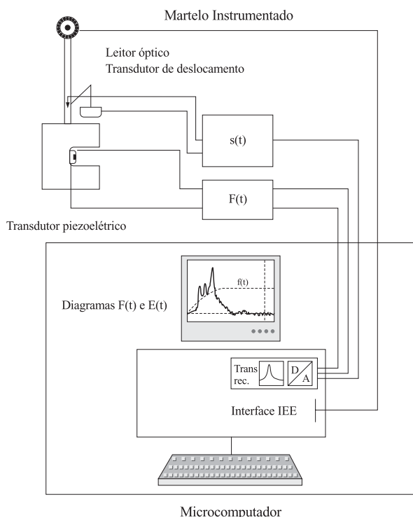
Figura 3. Diagrama esquemático do sistema de aquisição de dados no impacto instrumentado [2] .
