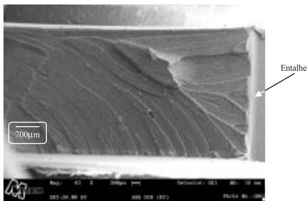
Figura 7. Superfície de fratura do ABS-810 após impacto à temperatura ambiente ilustrando fratura tipicamente dúctil.
