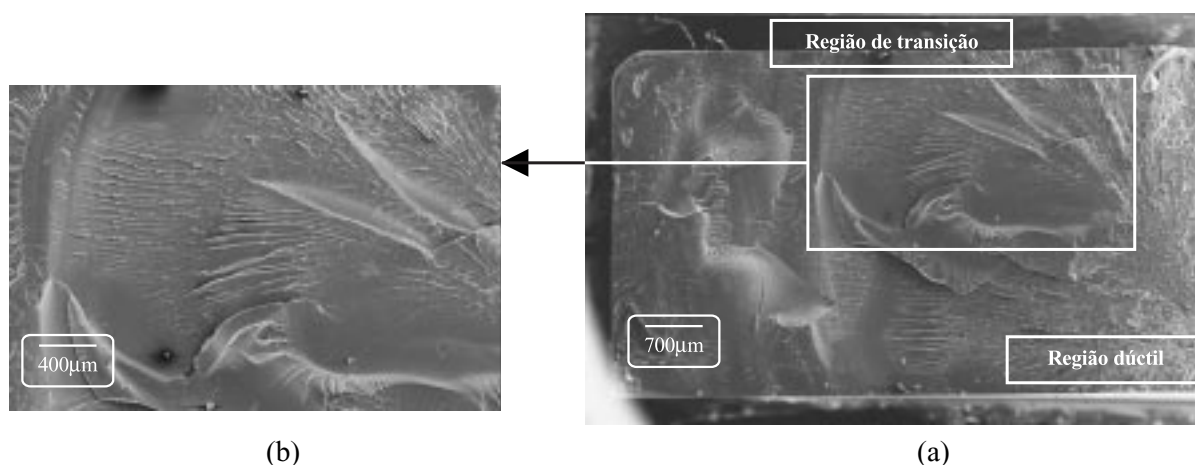
Figura 8. (a) Região de transição dúctil-frágil em superfície fraturada de amostra de ABS-810 após impacto à -60^{\circ}\text{C} . (b) Detalhe específico da região de transição.
