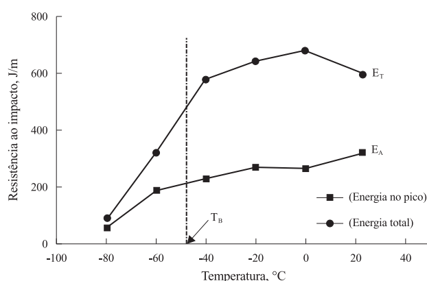
Figura 5. Resistência ao impacto do ABS ilustrando variação de energia na trinca e na fratura em função da temperatura. Izod – ASTM D256.
