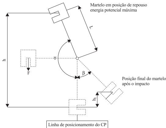
Figura 1. Princípio físico do pêndulo a martelo [2]
