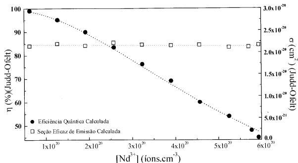
Figura 4. Eficiência quântica ( \eta ) e seção eficaz de emissão ( \sigma ) da transição {}^4F_{3/2} \rightarrow {}^4I_{11/2} (1076nm), em função da concentração de Nd^{3+} na matriz CASM. Os valores foram obtidos das equações 7 e 9.
