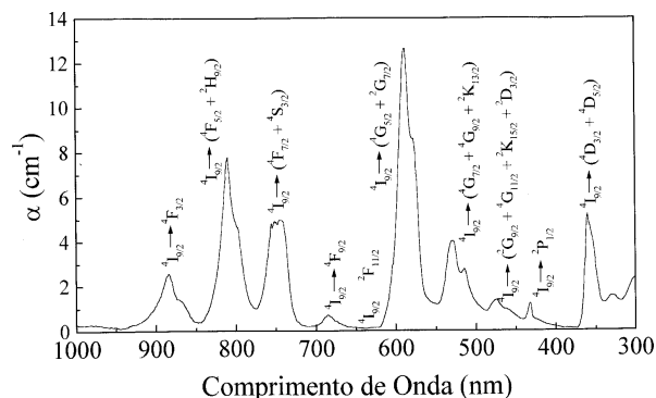
Figura 2. Espectro de absorção do vidro CASM contendo 5% de Nd 2 O 3 (amostra com 0,3cm de espessura, 300K).
