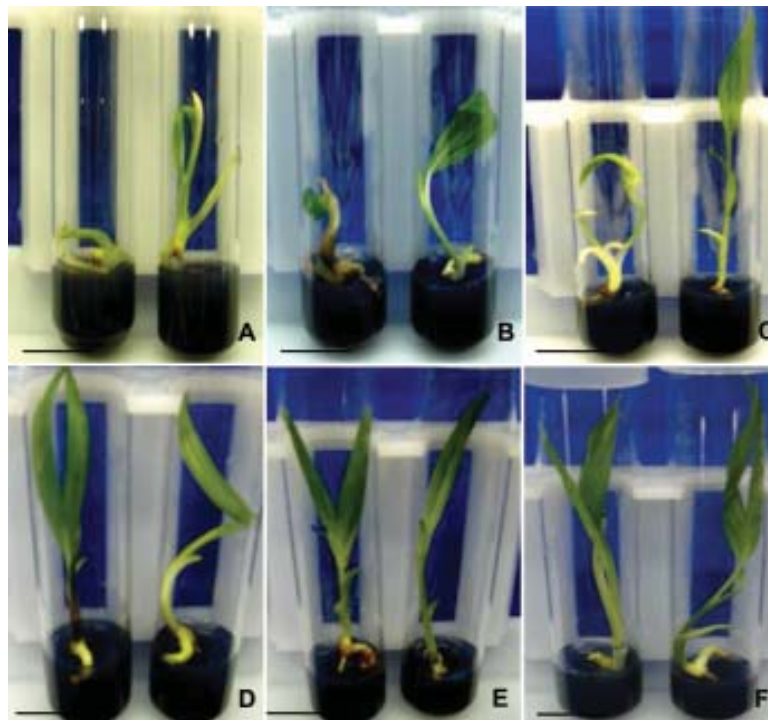
Figura 1 – Influência de temperaturas de armazenamento dos frutos (temperatura ambiente a 27 \pm 2 °C e câmara fria, a 12 a 15 °C) e sacarose (5, 10, 15, 20, 25 e 30 g L -1 ) na germinação in vitro de embriões zigóticos maduros de macaúba ( Acrocomia aculeata ). Plântulas obtidas após 90 dias da inoculação. A) 5 g L -1 de sacarose; B) 10 g L -1 de sacarose; C) 15 g L -1 de sacarose; D) 20 g L -1 de sacarose; E) 25 g L -1 de sacarose; F) 30 g L -1 de sacarose. Em A, B, C, D, E e F, à esquerda, plântulas obtidas de frutos armazenados à temperatura ambiente; e à direita de frutos armazenados em câmara fria, a 12-15 °C. (Barras = 20 mm).
