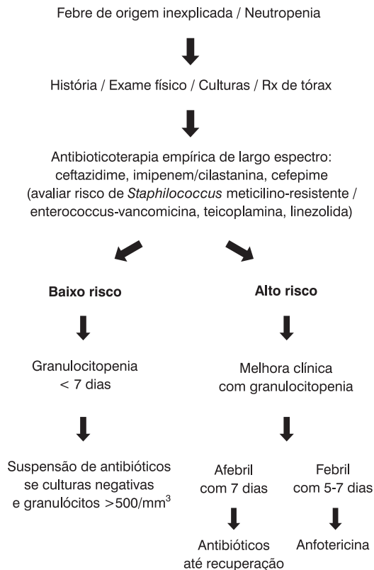
Figura 1 - Algoritmo para o tratamento inicial da criança neutropênica febril sem foco evidente. Modificado de Pizzo, A.P. 4
