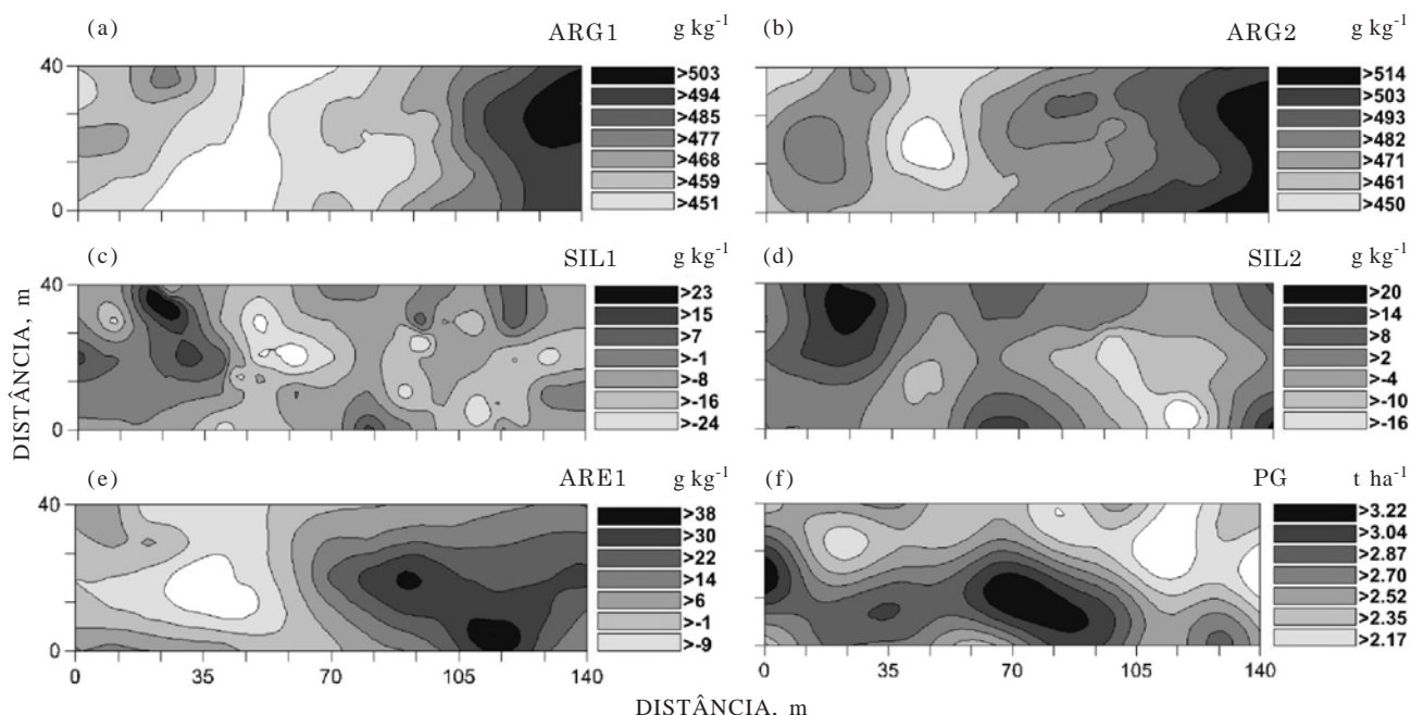
(a) ARG1: argila da camada 0,0–0,10 m; (b) ARG2: argila da camada 0,10–0,20 m; (c) SIL1: silte da camada 0,0–0,10 m; (d) SIL2: silte da camada 0,10–0,20 m; (e) ARE1: areia da camada 0,0–0,10 m, e (f) PG: produção de grãos do feijoeiro.
