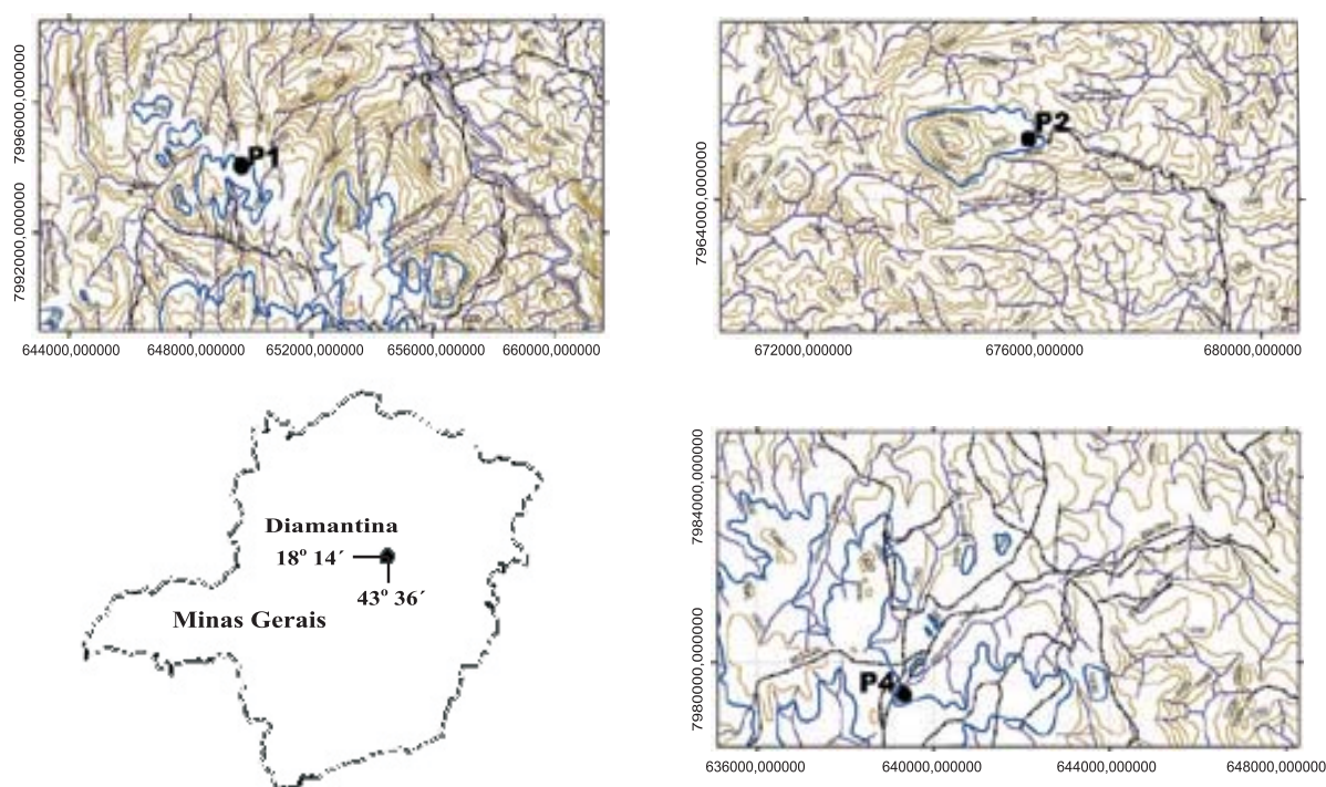
Figura 1. Localização das áreas de estudo. O mapa onde os perfis P1 e P4 estão localizados corresponde à carta topográfica Diamantina – Folha SE-23-Z-B-I e o mapa onde o perfil P2 está localizado corresponde à carta topográfica Rio Vermelho – Folha SE-23-Z-A-III, ambas na escala original de 1:100.000, digitalizadas utilizando o software Arc View 9.0.
