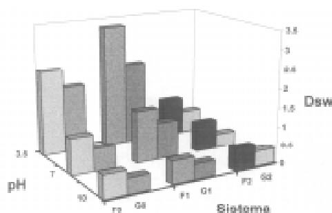
Figura 5. Perfil de intumescimento dos géis nos sistemas, Fo (formaldeído), Go (glutaraldeído), sem aditivos e aditivados com fenol (F1 e G1) e trihidroxibenzeno (F2 e G2) em sistemas tamponados após 24 horas.
