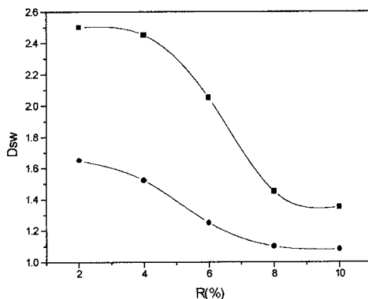
Figura 2. Variação do grau de intumescimento de géis de quitosana em função da concentração (R) do reticulante a pH 4,0, após 48 horas. (■ - Formaldeído ● - Glutaraldeído)
