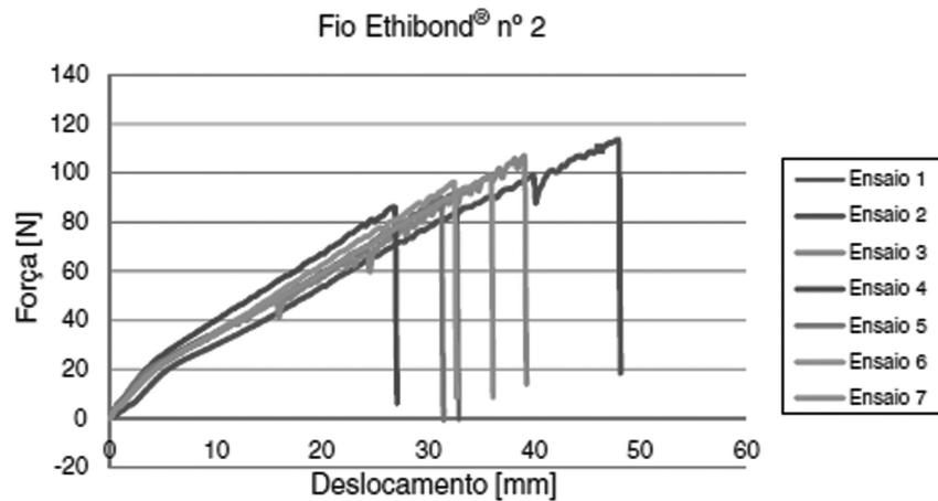
Fig. 4 Gráfico dos valores de força deformação dos ensaios do fio Ethibond® nº 2.
