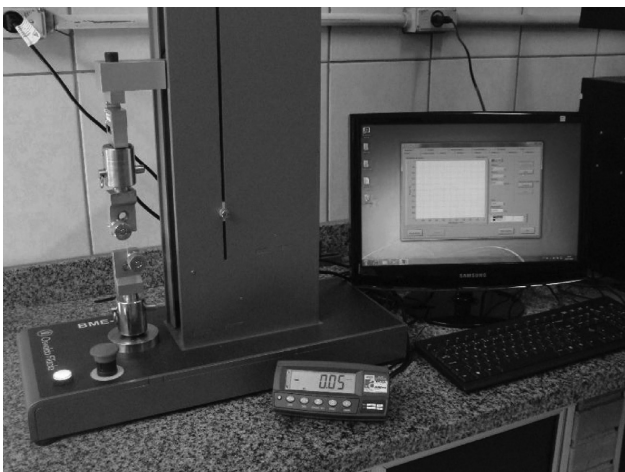
Fig. 2 Aparato experimental dos ensaios de tração: máquina de ensaios mecânicos BME 10 kN, célula de carga de 50 kgf e garras de fixação.
