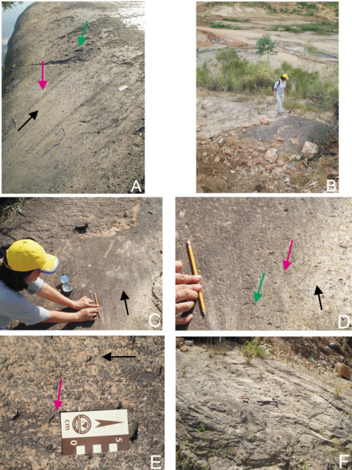
Figura 3 - Afloramentos onde há presença de superfícies estriadas (A1 e A2). A1 (A e E) e A2 (B, C e D), com orientação média das estrias N43°W (paralelas às setas pretas) e diamictitos do A2 (F); movimento das massas de gelo de SE para NW (setas pretas) atestado pela presença de finas fraturas com mergulhos para NW que cortam as estrias (setas vermelhas) e marcas de fricção (setas verdes).
