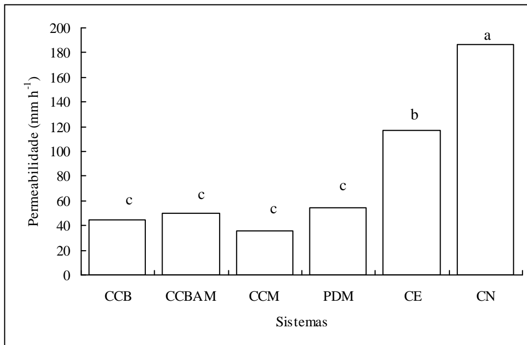
FIGURA 2 – Permeabilidade do solo à água em um Latossolo Vermelho-Amarelo Ácrico típico em diferentes sistemas de manejo. (CCB: Cultivo convencional de batata; CCBAM: Cultivo convencional de batata sucedido por aveia após uma subsolagem, e rotacionado com milho; CCM: Cultivo convencional com milho em rotação com feijão; PDM: Plantio direto com milho, após os cultivos convencionais com batata, arroz e milho; CE: Cultivo de eucalipto e CN: Cerrado nativo. Médias seguidas pela mesma letra não diferem estatisticamente entre si, pelo teste de Scott e Knott ao nível de 5% de probabilidade).
