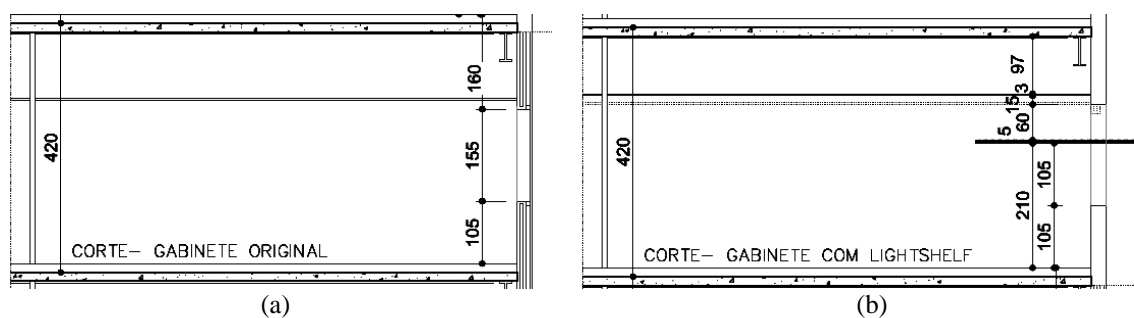
Figura 8 - Corte do ambiente em estudo mostrando em (a) o projeto original e em (b) as alterações que viabilizaram o uso de prateleira de luz ( lightshef )
