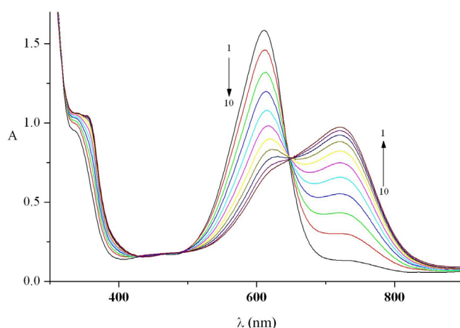
FIGURE 6 - UV-Vis spectra obtained for 1.0 \times 10^{-4} mol L -1 indigo carmine in 0.1 mol L -1 carbonate buffer solution at pH 10 in the presence of Cu(II) solutions: 1) 1.0 \times 10^{-5} ; 2) 2.0 \times 10^{-5} ; 3) 3.0 \times 10^{-5} ; 4) 4.0 \times 10^{-5} ; 5) 5.0 \times 10^{-5} ; 6) 6.0 \times 10^{-5} ; 7) 7.0 \times 10^{-5} ; 8) 8.0 \times 10^{-5} ; 9) 9.0 \times 10^{-5} and 10) 1.0 \times 10^{-4} mol L -1 .
