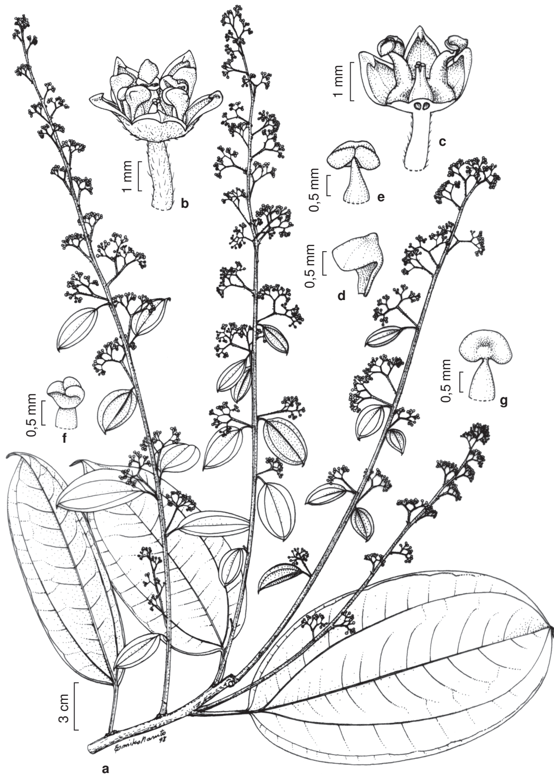
Figura 1 - Ampelozizyphus amazonicus : a. hábito; b. flor inteira; c. flor em corte longitudinal; d. pétala; e-g. estame (M. A. D. Souza & C. F. Silva 163).
