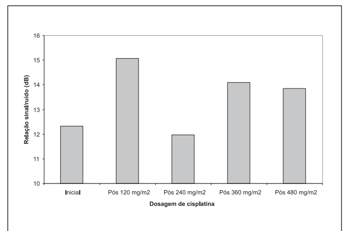
Gráfico 3. Valores médios da relação sinal/ruído (dB) da resposta global das EOAT por ciclo de cisplatina. (p=0,864)
