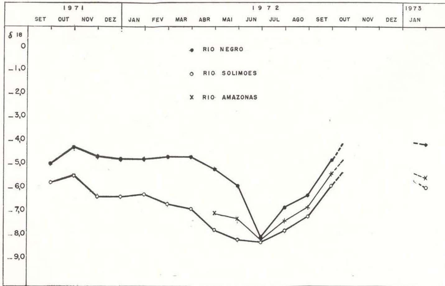
Fig. 2 — Variações de \delta 18 nos rios Negro (Manaus), Solimões (próximo de Manaus) e Amazonas (S. José do Amajari)
