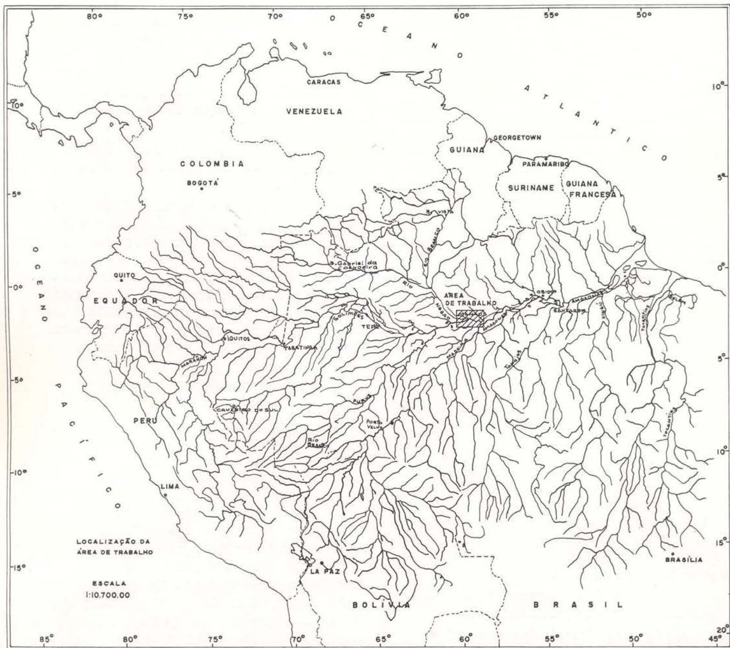
Fig. 1 — HIDROLOGIA ISOTÓPICA DA AMAZÔNIA — Vazões relativas dos rios Negro e Solimões através das concentrações de ^{18}O
