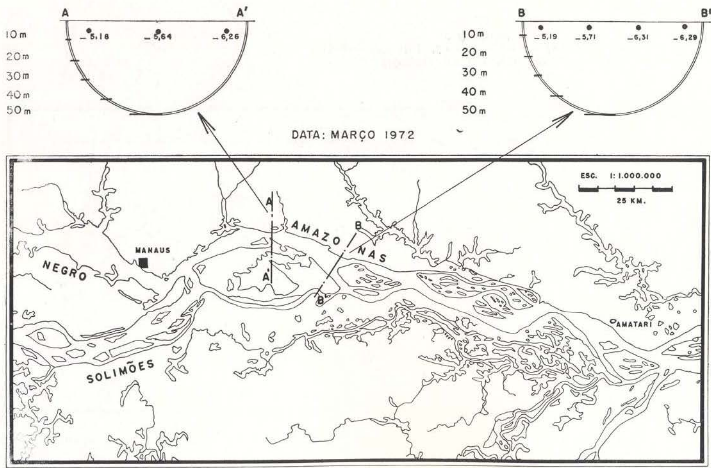
Fig. 3 — HIDROLOGIA ISOTÓPICA DA AMAZÔNIA — Concentrações de \delta^{18} em águas do rio Amazonas nos cortes indicados
