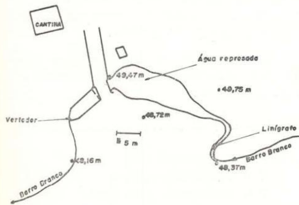
Fig. 1 — Detalhes do local de medição do escoamento superficial.
