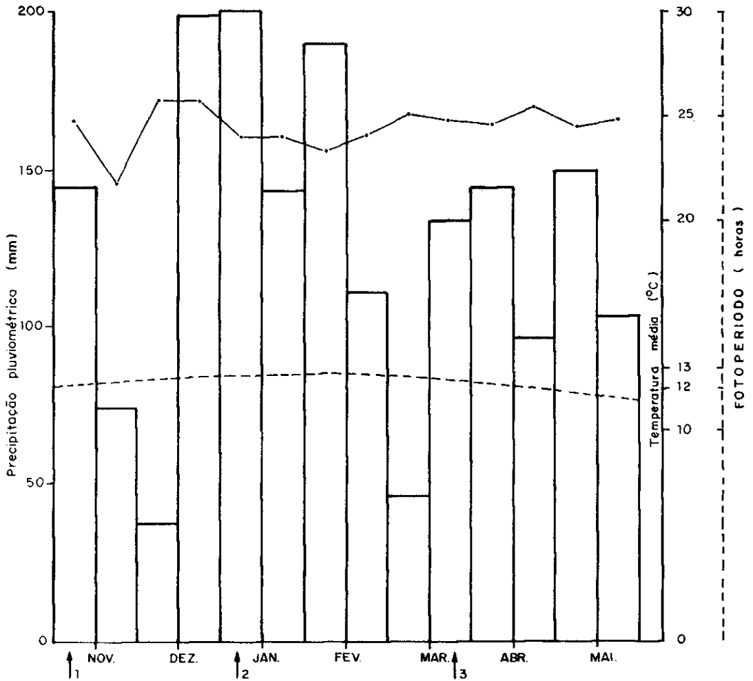
Figura 1. Distribuição do fotoperíodo, temperatura média e precipitação pluviométrica, acumulada por quinzenas, verificadas na Reserva Ducke/INPA (Manaus-AM, no período de NOVEMBRO/80 a MAIO/81. São indicadas as épocas de plantio (1), início do florescimento (2) e colheita inicial (3), do ensaio commomona
