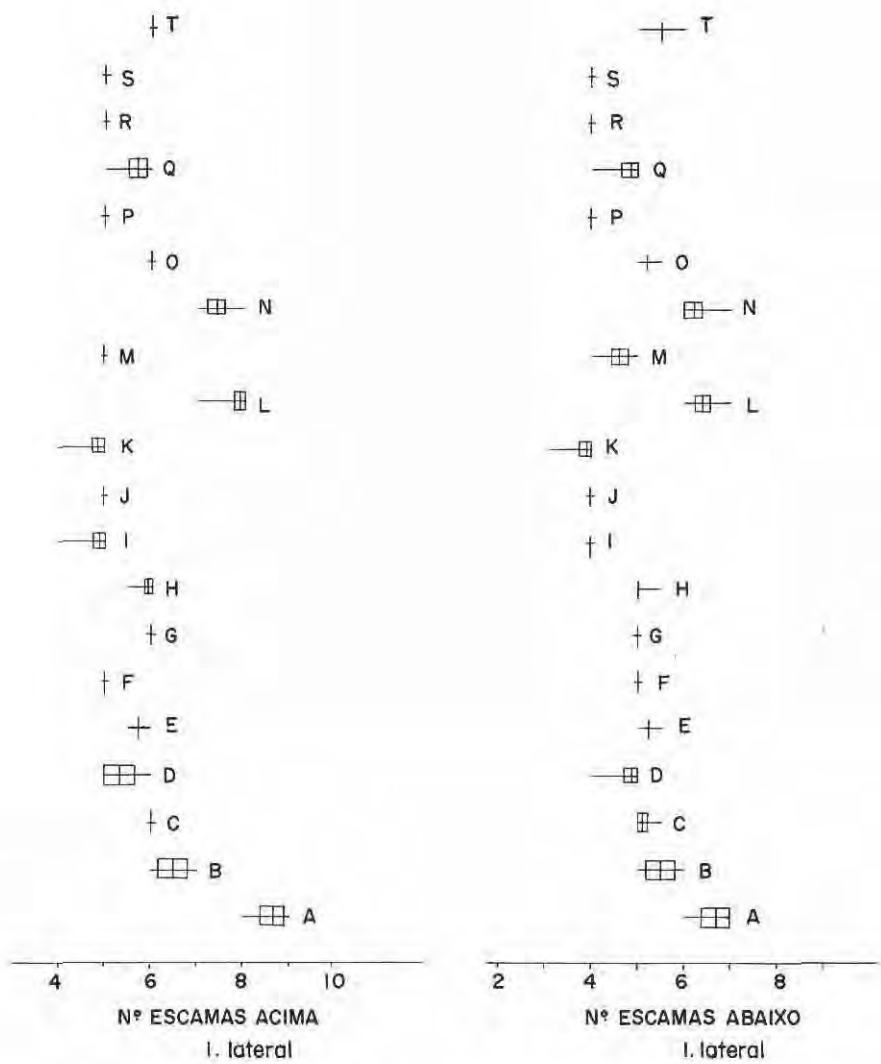
Fig. 4. Número de escamas acima e abaixo da linha lateral. A barra vertical em cada amostra indica a média; a barra horizontal a amplitude da variável e o retângulo, o erro padrão da média. Legenda na Fig. 2.
