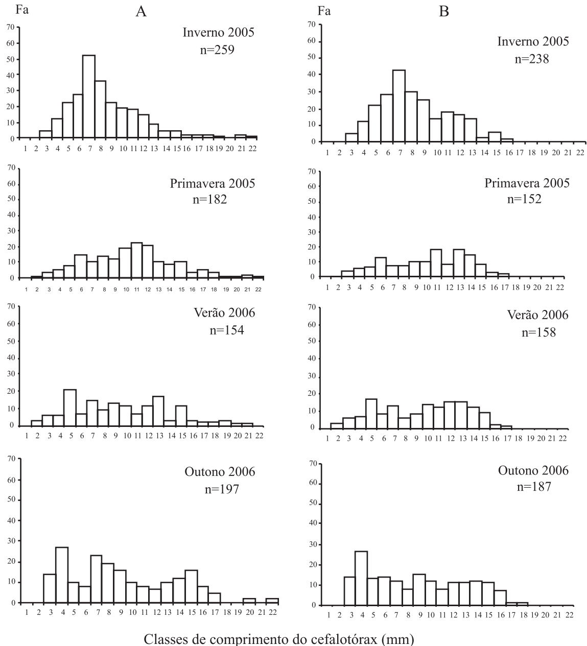
Figura 2. Distribuição das frequências absolutas sazonais do comprimento do cefalotórax (mm) de machos (A) e fêmeas (B) de Aegla itacolomiensis Bond-Buckup & Buckup, 1994, amostradas no período de junho de 2005 a maio de 2006 no arroio Solitária Alta, tributário da bacia hidrográfica do rio dos Sinos, RS. (1) = 0+1, (2) = 1+2, (3) = 2+3, (4) = 3+4, (5) = 4+5, (6) = 5+6, (7) = 6+7, (8) = 7+8, (9) = 8+9, (10) = 9+10, (11) = 10+11, (12) = 11+12, (13) = 12+13, (14) = 13+14, (15) = 14+15, (16) = 15+16, (17) = 16+17, (18) = 17+18, (19) = 18+19, (20) = 19+20, (21) = 20+21, (22) = 21+22. Fa = Frequência absoluta de indivíduos.
