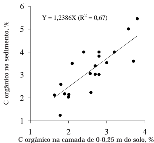
Figura 2. Relação do carbono orgânico contido na camada de 0-0,025 m de profundidade do solo e no sedimento da erosão hídrica, em três ciclos culturais num Cambissolo Húmico aluminico (média da rotação e sucessão de culturas).
