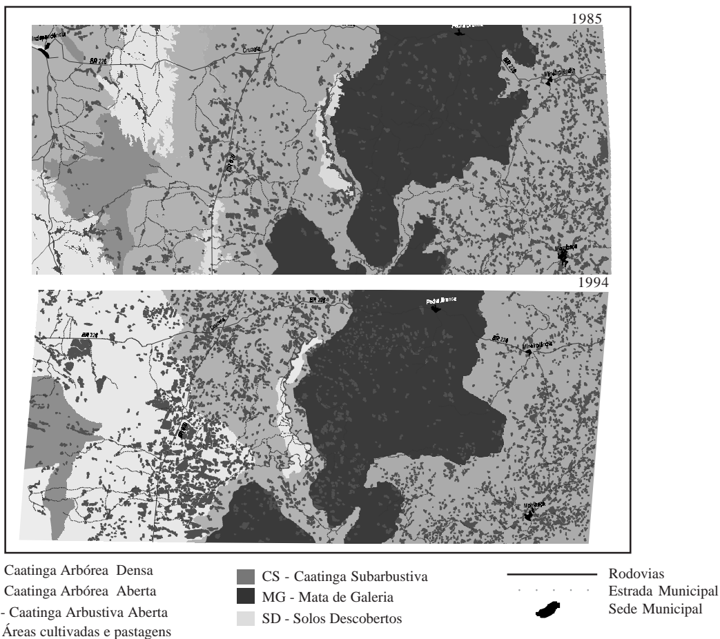
Figura 2. Sobreposição das cartas de vegetação e áreas cultivadas e pastagens (interpretação a partir da imagem Landsat TM-5, WRS 217/064A; passagens em 20 de julho de 1985 e 14 de agosto de 1994).
