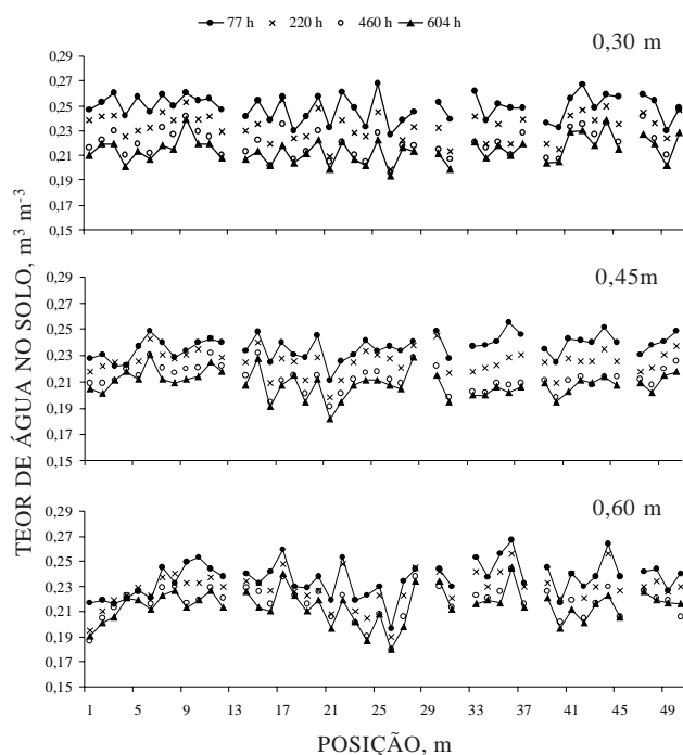
Figura 2. Variabilidade do teor de água no solo ( m^3 m^{-3} ), segundo uma transeção de 50 pontos espaçados de um metro, em três profundidades e quatro tempos de amostragem. A linha interrompida indica os cinco pontos de medida que foram eliminados.
