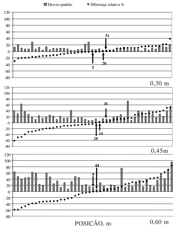
Figura 5. Diferença relativa média intertemporal e desvio-padrão para o potencial mátrico da água no solo (kPa), em três profundidades, segundo uma transeção de 50 pontos espaçados de um metro. Valores em destaque indicam os pontos que devem ser adotados para medidas representativas da média de potencial mátrico do solo.
