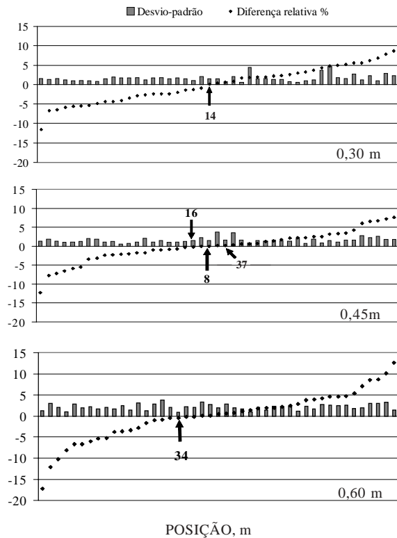
Figura 4. Diferença relativa média intertemporal e desvio-padrão para o teor de água no solo ( m^3 m^{-3} ), em três profundidades, segundo uma transeção de 50 pontos espaçados de um metro. Valores em destaque indicam os pontos que devem ser adotados para medidas representativas da média de umidade no solo.
