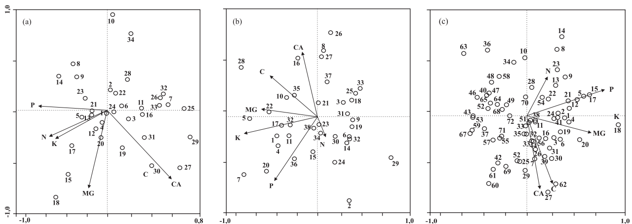
Figura 2. Diagrama de ordenação produzido pela análise de componentes principais do teor de nutrientes e carbono em folhas de espécies encontradas em fragmentos florestais da Mata Atlântica, na região norte-fluminense. (a) fragmento M1; (b) fragmento M2; e (c) fragmentos M1 (espécies de nº 1 a 34) e M2 (espécies de nº 35 a 72).
