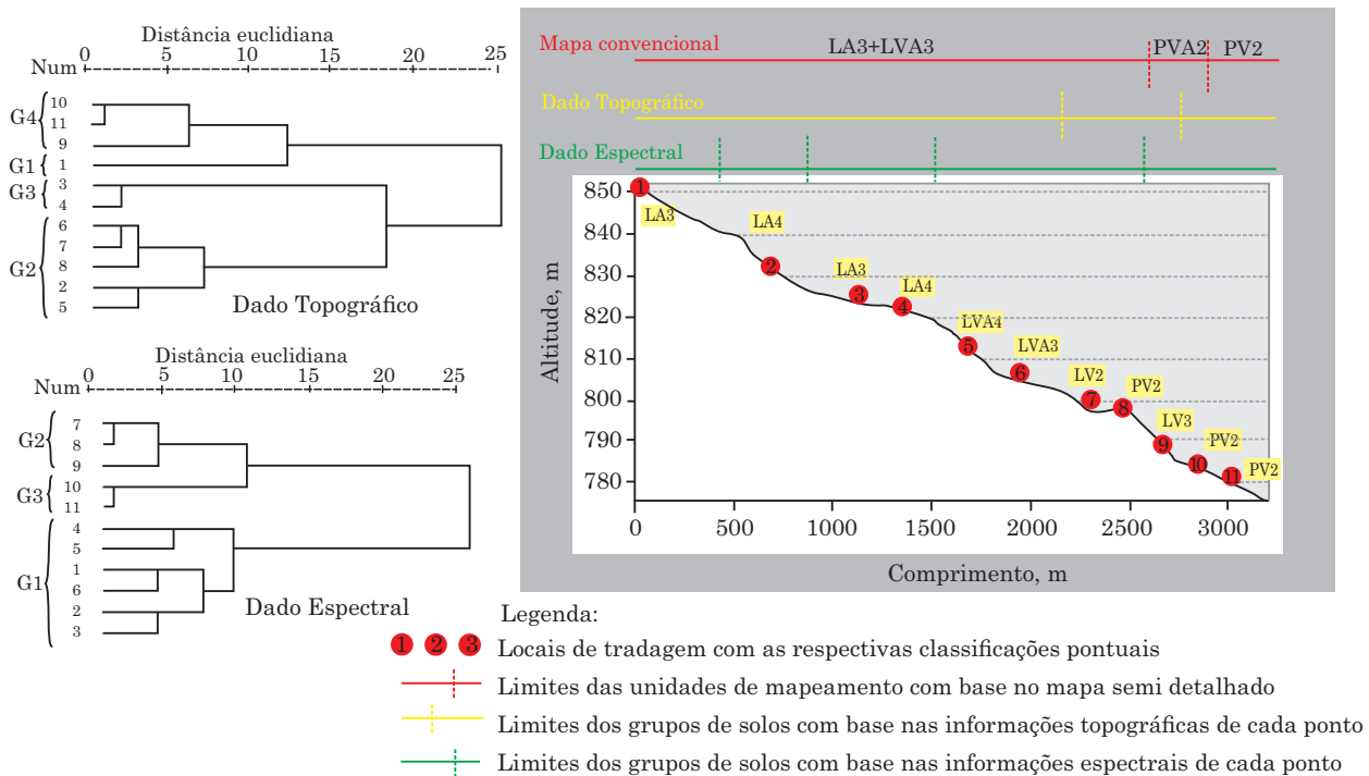
Figura 2. Representação gráfica da Toposequência 1 com as respectivas classificações pedológicas e os dendrogramas das inter-relações dos 11 pontos referentes aos atributos topográficos e espectrais.
