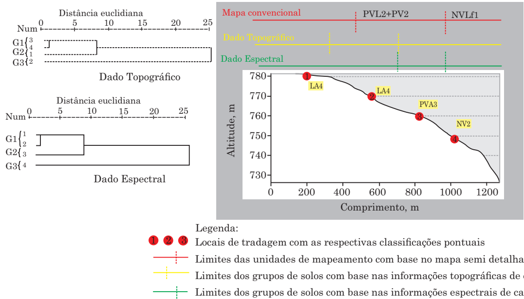
Figura 3. Representação gráfica da Toposequência 5 com as respectivas classificações pedológicas e os dendrogramas das inter-relações dos quatro pontos referentes aos atributos topográficos e espectrais.
