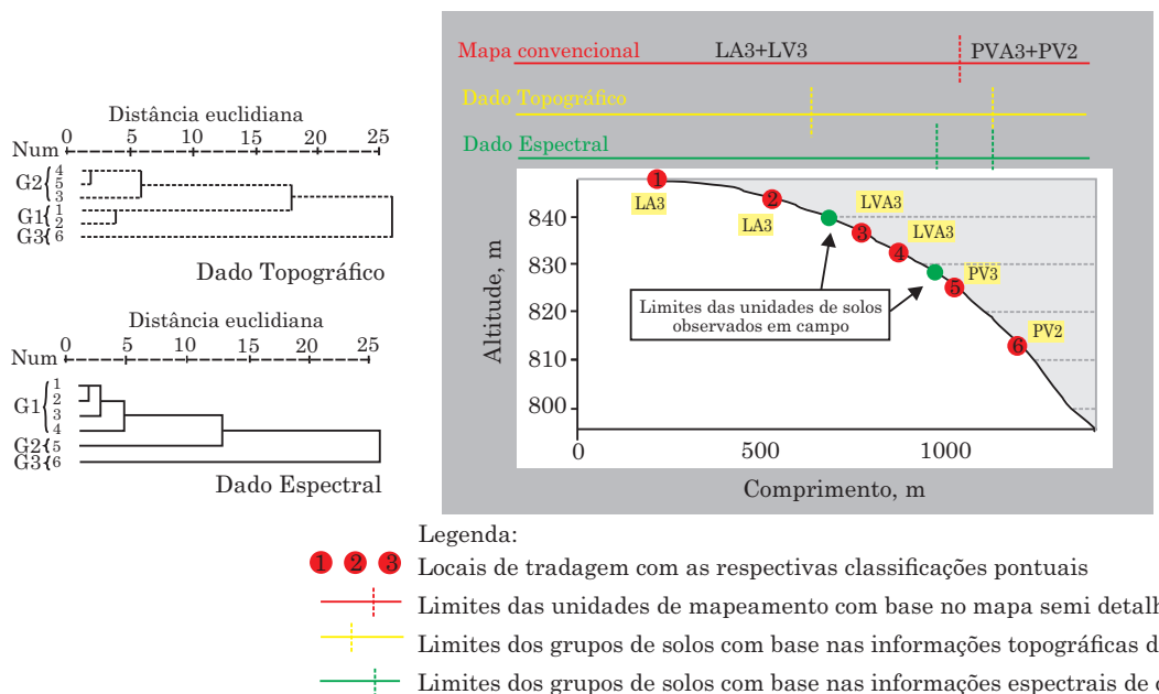
Figura 4. Representação gráfica da Toposequência 12 com as respectivas classificações pedológicas e os dendrogramas das inter-relações dos seis pontos referentes aos atributos topográficos e espectrais.
