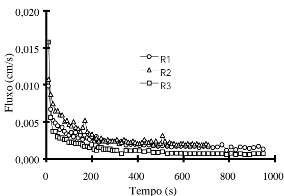
FIG. 2. Evolução do fluxo com o tempo para três repetições (R1, R2 e R3), na profundidade de 70 cm, potencial de fornecimento -5 cm e raio do disco permeâmetro de 12,5 cm.
