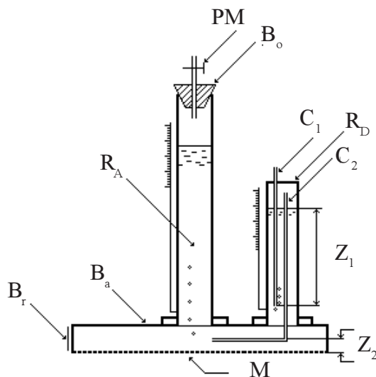
FIG. 1. Esquema do permeâmetro a disco. B_a , base de contato com o solo; M , membrana constituída por uma tela de tecido de náilon (abertura 20 \mu\text{m} ) presa por um bracelete de borracha ( B_r ); R_A , reservatório de alimentação fechado no seu topo por uma rolha de borracha ( B_o ) na qual está acoplado um pequeno tubo munido de um duto flexível e de uma pinça de Mohr ( PM ); R_D , reservatório lateral de depressurização; C_1 , tubo capilar para regular o valor do potencial de fornecimento de água ao nível de membrana; C_2 , que realiza a comunicação entre este reservatório e a base do permeâmetro.
