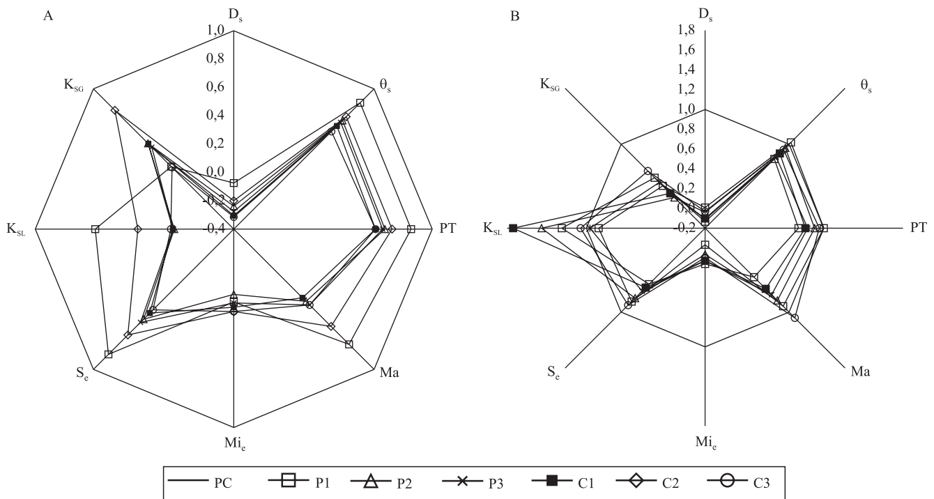
Figura 2. Diagrama comparativo da qualidade física do solo de áreas sob diferentes sistemas de manejo e uso, na profundidade 0–20 cm, para A, 2005 e B, 2006. D_s , densidade do solo; \theta_s , umidade gravimétrica do solo na amostragem; PT, porosidade total do solo; Ma, macroporosidade; Mi_e , microporosidade efetiva; S_e , saturação efetiva; K_{SL} , condutividade hidráulica saturada de laboratório; K_{SG} , condutividade hidráulica saturada de campo; PC, pastagem contínua, com 19 anos de uso; P1, pastagem de Urochloa brizantha , com quatro anos de uso; P2, pastagem de U. brizantha , com dois anos de uso; P3, pastagem de U. brizantha , com três anos de uso; C1, soja sob plantio direto; C2, arroz em plantio convencional; C3, U. brizantha em consórcio com milho.
