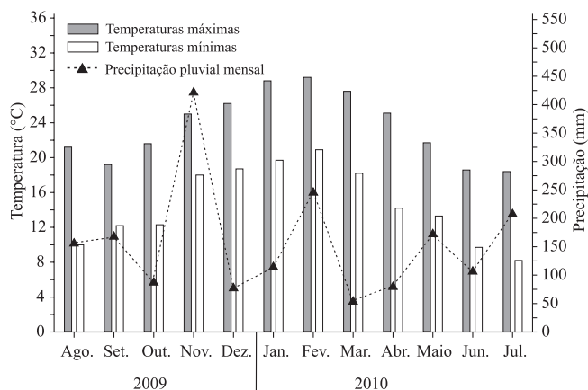
Figura 1. Médias mensais das temperaturas máximas e mínimas e totais da precipitação pluvial mensal de agosto a julho, no ciclo 2009/2010. Capão do Leão, RS, 2010.
