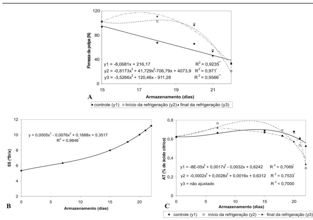
FIGURA 2 - Firmeza da polpa (A), teor de sólidos solúveis – SS – (B) e acidez titulável - AT – (C) de manga ‘Tommy Atkins’ submetida a diferentes épocas de aplicação de 1-MCP e armazenada sob refrigeração ( 10,6^{\circ}\text{C} \pm 3,6 e 84\% \text{ UR} \pm 7 ) durante 15 dias, seguidos de até 7 dias em temperatura ambiente ( 24,4^{\circ}\text{C} \pm 2,9 e 42\% \text{ UR} \pm 11 ). Em B, estão representados os valores médios das épocas de aplicação de 1-MCP.
