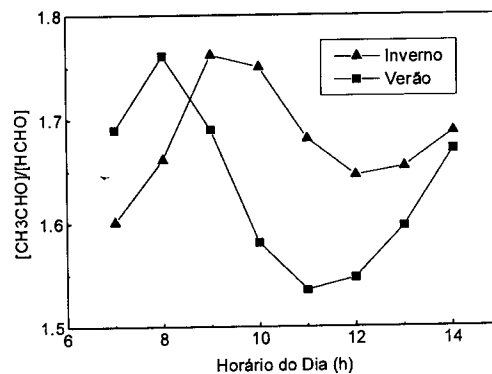
Figura 7. Relação [CH_3CHO]/[HCHO] calculada com o modelo completo para o inverno e verão.
