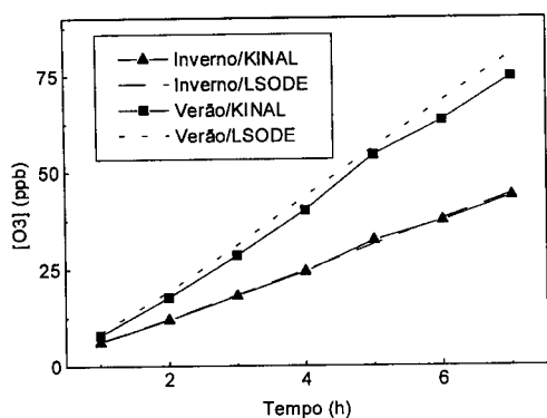
Figura 4. Modelagem da evolução temporal das concentrações de O_3 sem emissões veiculares, com acetaldeído e formaldeído, no verão e no inverno, nas condições do modelo.
