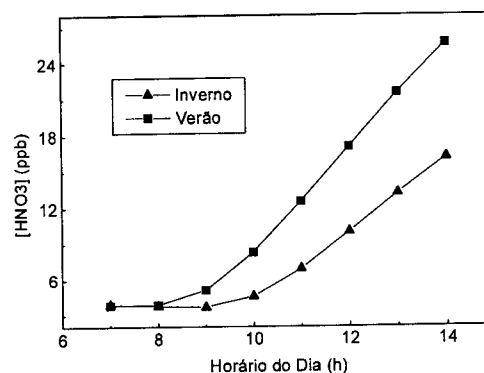
Figura 8. Concentrações de HNO_3 calculadas com o modelo completo para o verão e o inverno.
