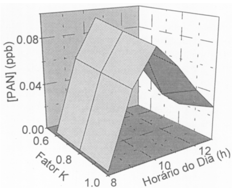
Figura 11. Concentração de PAN em função do horário do dia e concentração de NO (Fator K) calculada com o modelo completo para o verão. K igual a 1.0 refere-se a uma emissão de NO de 12 ppb/h.
