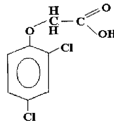
Figura 1. Fórmula Estrutural do Herbicida 2,4 D (Ácido 2,4 Diclorofenoxiacético).
