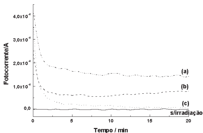
Figura 3. Fotocorrentes dos sistemas ITO-TiO 2 em soluções aquosas contendo (a) Na 2 SO 4 , (b) KCl ou (c) KI 0,1 mol L -1 , com potencial aplicado de 0,20 V. T = 298 K. Área do eletrodo = 4,65 cm 2 e massa de TiO 2 = 3,20 mg
