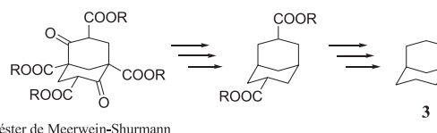
Figura 4. Representação simplificada da síntese do adamantano partindo de éster de Meerwein-Schurmann
