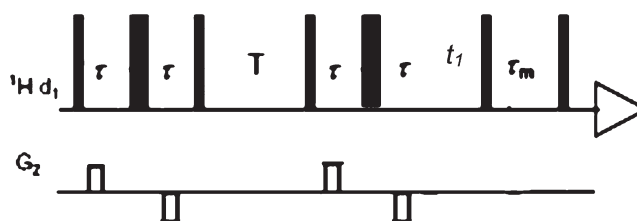
Esquema 6. Sequência de pulsos do experimento de DOSY-NOESY. Este experimento é uma junção da sequência STE com a sequência de NOESY. Os tempos t_1 e \tau_m são os tempos de evolução e de mistura, respectivamente
