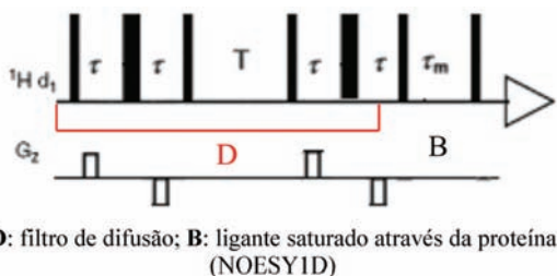
Esquema 4. a) Sequência de pulsos do experimento de WaterLOGSY. O sinal da água é seletivamente invertido em varreduras alternadas de pulsos de 90° e deslocamentos de fase dos pulsos seletivos de 180°. A transferência de magnetização da água invertida, tanto para os ligantes livres como ligados, ocorre durante o T_m ; b) mecanismos de transferência de magnetização fundamentais do WaterLOGSY. A transferência de magnetização a partir da água para os ligantes ocorre via hidrogênios lábeis do receptor dentro e fora do sítio ativo. As bolinhas azuis indicam as moléculas de água invertidas. Somente os ligantes ligados experimentam ambos tipos de transferência de magnetização
