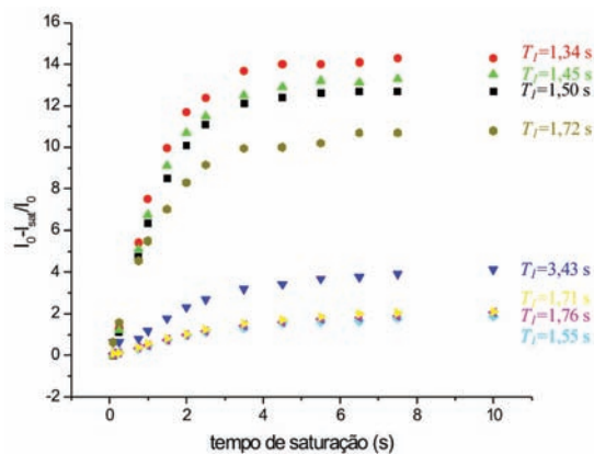
Figura 2. Gráfico do fator STD (%) versus o tempo de saturação (s) para mistura 1 . A proteína foi irradiada com um trem de pulsos Gaussianos em -0,50 ppm para o espectro de STD e em 30 ppm para o espectro de STD-control. Os espectros foram adquiridos com um d_1 = 1 s e o tempo de saturação foi ajustado pelo número de pulsos Gaussianos. O tempo de relaxação longitudinal ( T_1 ) para cada sinal na presença de BSA (● H-4, ▲ H-3,5 e ■ H-6 de (1); ▼ H-8, ► CH 3 -1, ◄ CH 3 -3, ◆ CH 3 -9 de (2) e ● TPSA) está apresentado no gráfico
