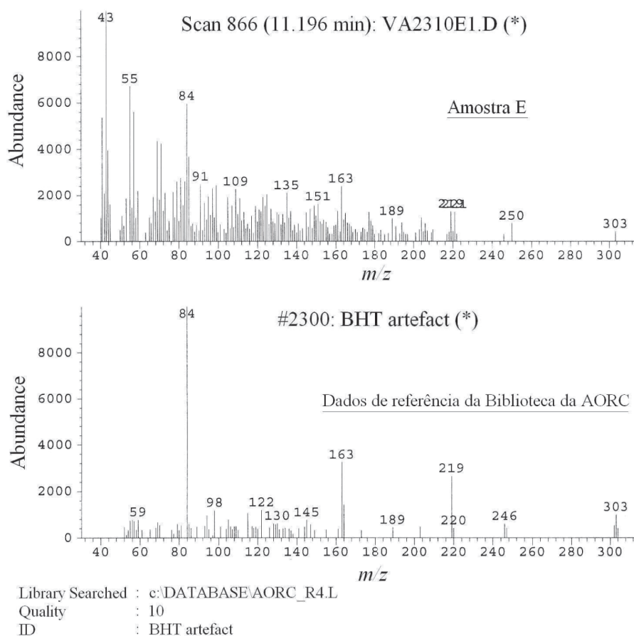
Figura 1S. Espectro de massas relativo à amostra E e sua comparação com dados de referência da base de dados da Biblioteca da Association of Official Racing Chemists (AORC)
