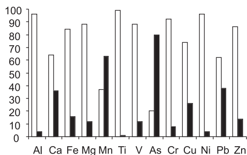
Figura 1. Porcentagem de elementos químicos na fração residual do solo (□) e nas demais frações (solúvel, trocável, orgânica e óxidos de Al, Fe e Mn) denominada de porcentagem parcial (■)
