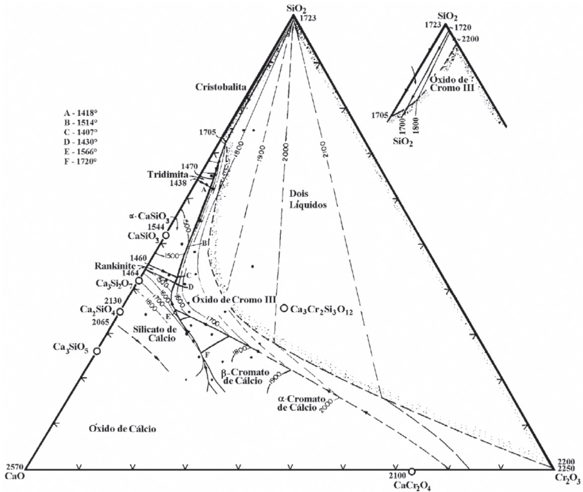
Figura 2S. Diagrama ternário \text{CaO-Cr}_2\text{O}_3\text{-SiO}_2 , adaptado da ref. 3.
