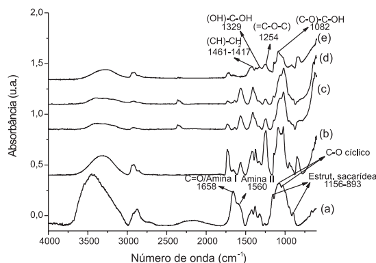
Figura 1. Espectros de IV dos filmes de quitosana pura (a) e blenda Q/P (3:1) (b); Q/P (1:1) (c); Q/P (1:3) (d); e PVA puro (e)
