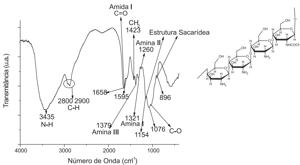
Figura 2S. Espectro de IV típico da quitosana (GD=75,6%) e estrutura química da quitosana parcialmente desacetilada
