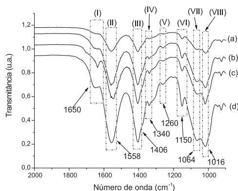
Figura 2. Espectros de IV dos filmes de quitosana pura (a) e reticulados com 0,5% (b); 1,0% (c) e 5,0% (d) de GA
