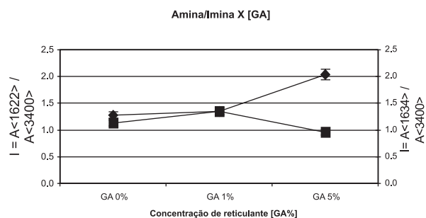
Figura 3. Evolução das bandas de formação de imina (C=N) e redução de amina (NH 2 ), durante a reticulação da quitosana pelo GA na blenda Q/P(1:3)
