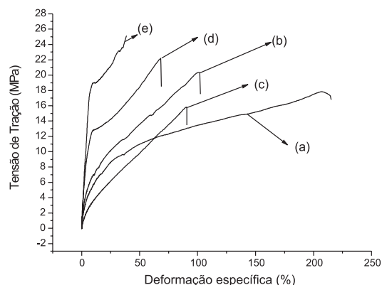
Figura 5. Gráfico de tensão x deformação apresentando as curvas dos filmes sem reticulação de PVA(a), Q/P(1:3)(b), Q/P(1:1)(c), Q/P(3:1)(d) e quitosana(e)
