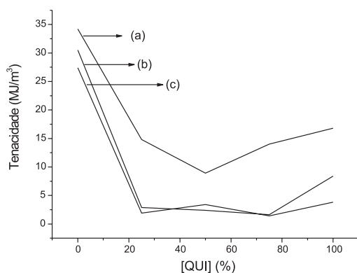
Figura 6. Influência da concentração de quitosana na tenacidade das blendas. Sem GA(a), 1% de GA(b) e 5% de GA(c)
