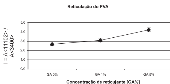
Figura 4. Evolução da banda de 1110 cm -1 durante a reticulação do PVA
