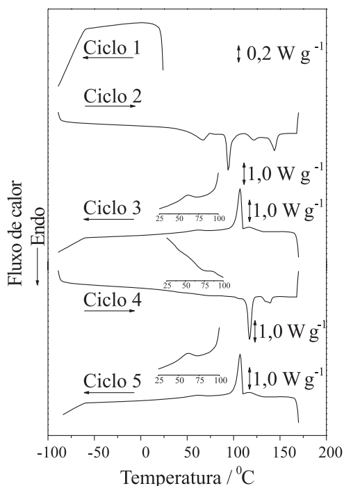
Figura 3. Curvas DSC do Napal, realizadas em ciclos de aquecimento/resfriamento entre -90 e 170\text{ }^{\circ}\text{C} com razão de resfriamento/aquecimento de 10\text{ }^{\circ}\text{C min}^{-1} , massa de amostra de 2\text{ mg} , atmosfera dinâmica de \text{N}_2 (vazão de 50\text{ mL min}^{-1} ). Síntese feita em meio etanólico. Nos detalhes, ampliação dos eventos observados em torno de 70\text{ }^{\circ}\text{C}
