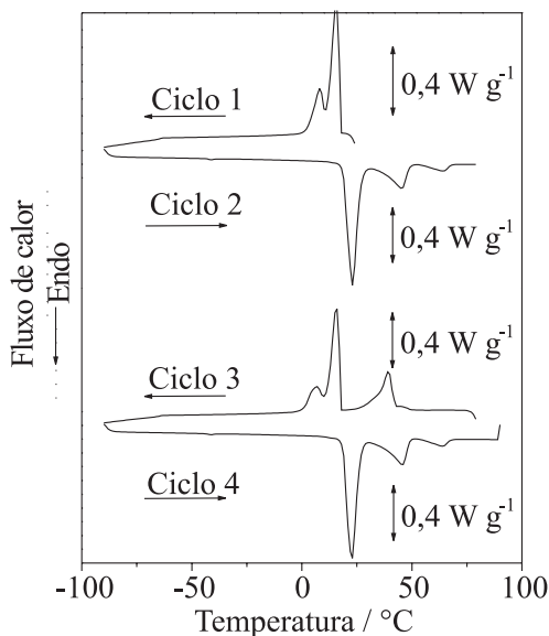
Figura 4. Curva DSC do palmitato de etila realizada em ciclos de aquecimento/resfriamento entre -90 e 170\text{ }^{\circ}\text{C} , com razão de resfriamento/aquecimento de 10\text{ }^{\circ}\text{C min}^{-1} , massa de amostra de 2\text{ mg} , atmosfera dinâmica de \text{N}_2 (vazão de 50\text{ mL min}^{-1} ).
