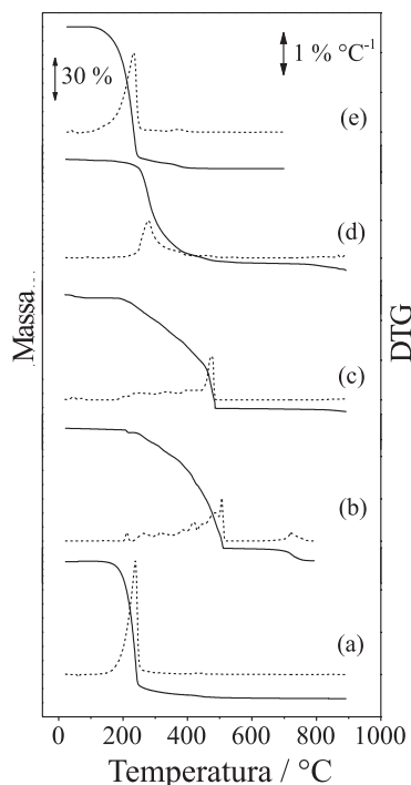
Figura 1. Curvas TG/DTG obtidas em razão de aquecimento de 10\text{ }^{\circ}\text{C min}^{-1} , atmosfera dinâmica de ar (vazão de 100\text{ mL min}^{-1} ), massa de amostra em torno de 3\text{ mg} , utilizando suporte de amostra aberto de alumina. (a) Hpal, (b) Lipal, (c) Napal, (d) Kpal e (e) Etílpal
