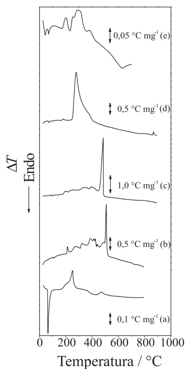
Figura 2. Curvas DTA obtidas em razão de aquecimento de 10\text{ }^{\circ}\text{C min}^{-1} , atmosfera dinâmica de ar (vazão de 100\text{ mL min}^{-1} ), massa de amostra em torno de 3\text{ mg} , utilizando suporte de amostra aberto de alumina. (a) Hpal, (b) Lipal, (c) Napal, (d) Kpal e (e) Etílpal
