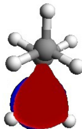
Figura 4S. Orbitais LUMO do 1-cloropropano
