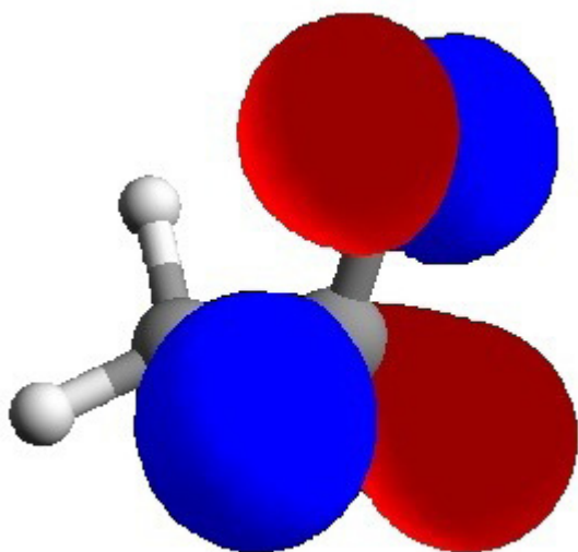
Figura 1S. Orbitais HOMO do íon etóxido
