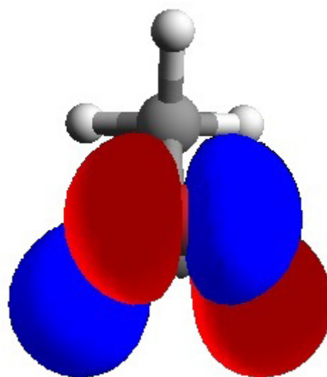
Figura 3S. Orbitais HOMO do íon etóxido
