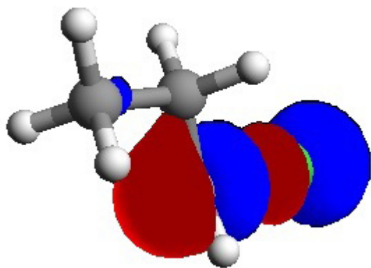
Figura 2S. Orbitais LUMO do 1-cloropropano
