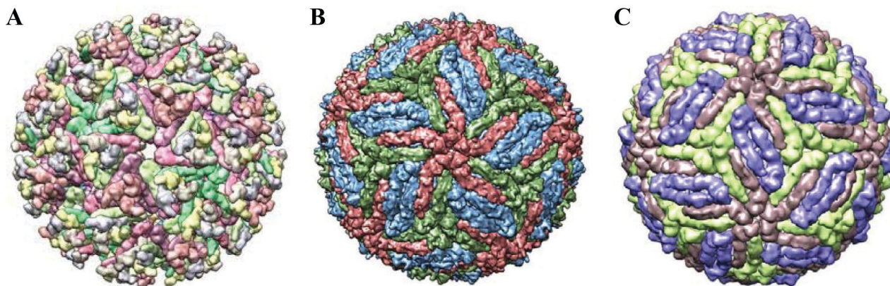
Figura 2. Estrutura 3D do envelope dos vírus (A) Chikungunya (PDB ID, 3J2W), 11 (B) Zika (PDB ID, 5IRE) 12 e (C) Febre do Oeste do Nilo (PDB ID, 3J0B) 13
