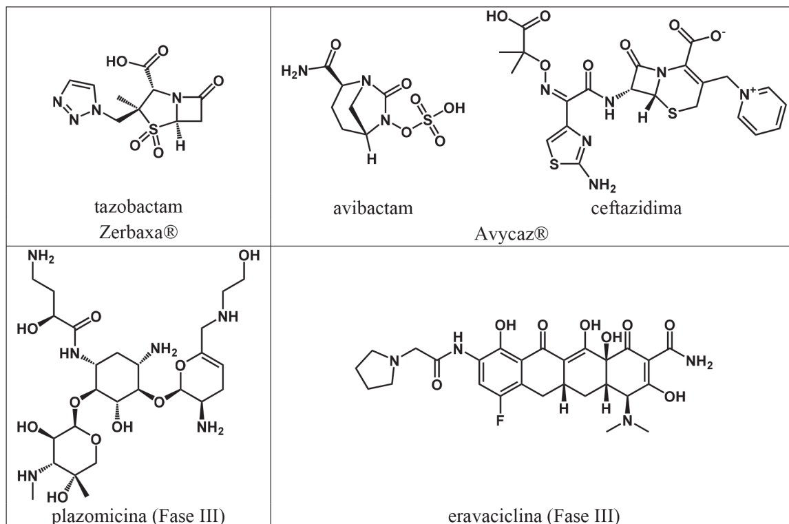
Figura 1. Estruturas químicas de novos fármacos aprovados e candidatos a fármacos em estudos avançados de Fase III para o combate de bactérias Gram-negativas da classe multirresistentes (MDR) e extensivamente resistentes (XDR)
