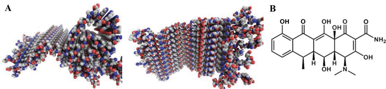
Figura 3. (A) Visão ortogonal da estrutura da \alpha -sinucleína obtida por RMN de estado sólido (PDB ID, 2N0A). (B) Estrutura molecular da doxiciclina
