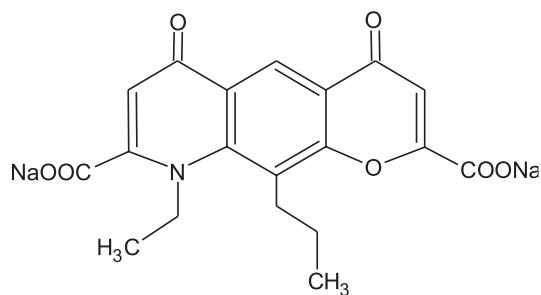
Figura 1. Fórmula Estrutural do Nedocromil de Sódio
