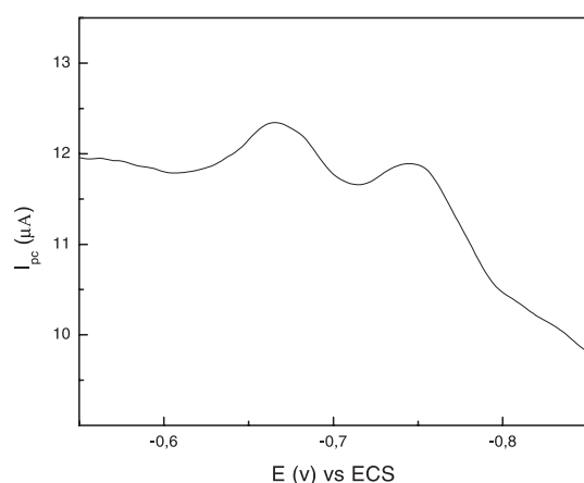
Figura 4. Voltamograma de pulso diferencial de solução 1,0 \times 10^{-5} mol L -1 de Nedocromil de Sódio em tampão B-R (pH 4,0); \Delta E_p = 100,0 mV; t_p = 10,0 ms; v = 5,0 mV s -1 .
