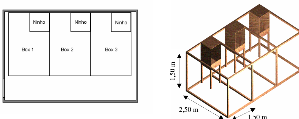
FIGURA 1. Esquema da construção e disposição dos boxes dentro da câmara climática.
