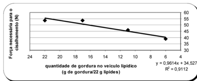
FIGURA 3 - Influência da redução progressiva da quantidade de gordura vegetal hidrogenada no veículo lipídico sobre a força necessária para o cisalhamento dos salgadinhos
