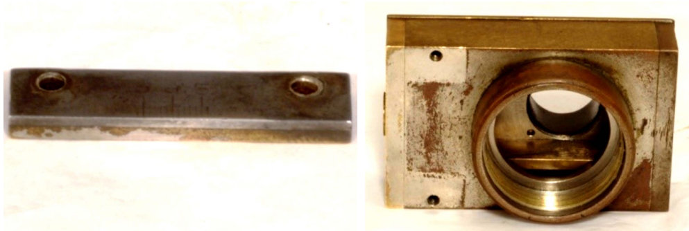
Figuras 13a (Sulcos perdidos na graduação da régua do micrômetro) e 13b (Liga de base exposta na câmera do micrômetro) – Danos provocados por uso recorrente de massa polidora. Fotos: Ricardo Dias, 2013.
